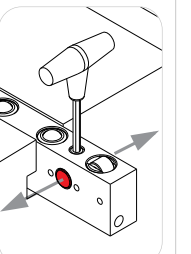
Seitliche Blockierung : BL
