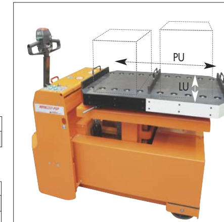
Tisch für 2 Werkzeuge mit einziehbaren Kugeln
