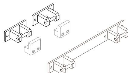
Werkzeughaken - Andocken
