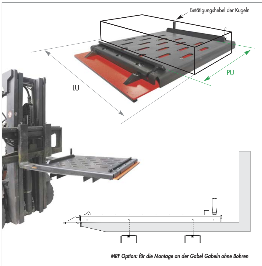
versenkte Kugeln: rutschfest
